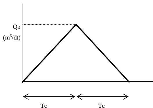
a. Durasi hujan &lt; waktu konsentrasi (Tc)
