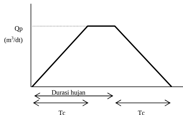
b. Durasi hujan &gt; waktu konsentrasi (Tc)
