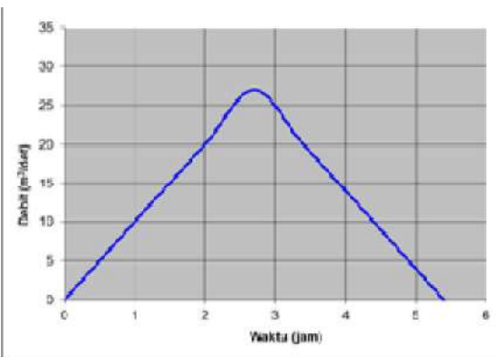
Gambar 7. Hidrograf Banjir Rancangan Kala Ulang 25 Tahun
