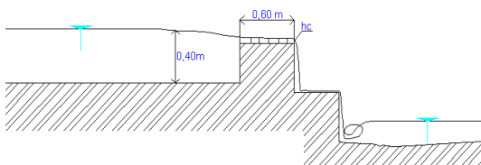
Gambar 2.b : Potongan Memanjang Aliran pada Bangunan Terjunan
