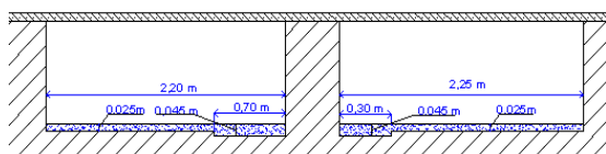
Gambar 2. a : Potongan melintang aliran sungai pada Bangunan Terjunan
