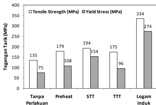
Gambar 12. Diagram perbandingan hasil uji tarik.
