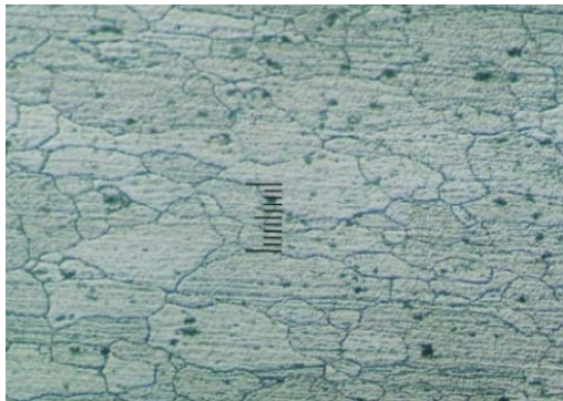
Gambar 9. Struktur mikro daerah logam induk ( base metal ).
