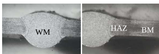
Gambar 6. Kampuh las.
