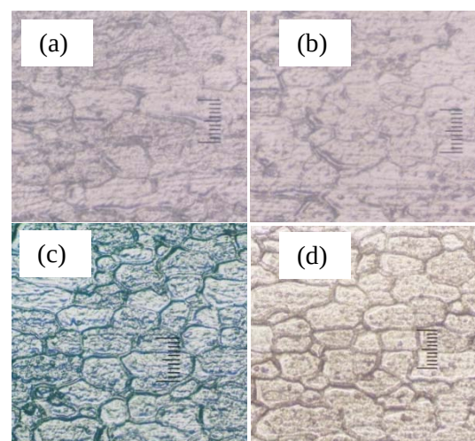
Gambar 8. Struktur mikro daerah HAZ : (a) tanpa perlakuan, (b) preheat 200°C, (c) STT 200°C, (d) TTT 200°C.
