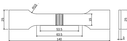
Gambar 5. Spesimen uji tarik berdasarkan JIS Z2201 no. 6.
