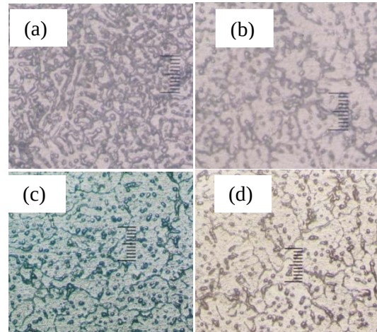
Gambar 7. Struktur mikro daerah las : (a) tanpa perlakuan, (b) preheat 200°C, (c) STT 200°C, (d) TTT 200°C.
