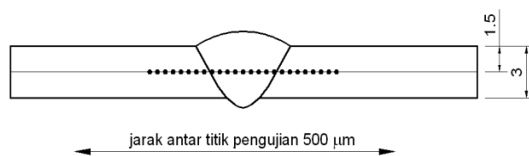
Gambar 4. Posisi Pengujian kekerasan.
