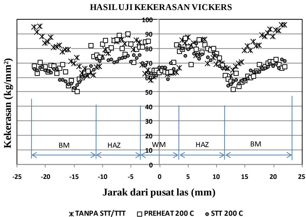
Gambar 10. Hasil pengujian kekerasan Vickers.
