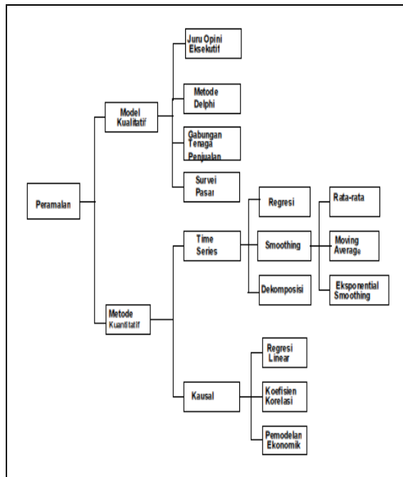
Gambar 1. Taksonomi Peramalan
