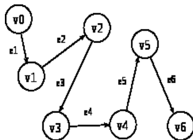
Gambar 3. Graf Berarah
