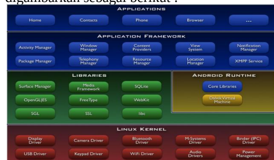
Gambar 4. Arsitektur Android
